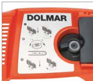
Beznástrojové napínání řetězu (TLC) u PS32CTL35B pro pohodlné napínání řetězu
